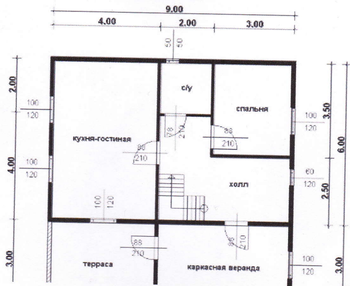
Схема первого этажа дома, размером 6,0х9,0 м + (3,0х5,0) м - каркасная веранда + (3,0х4,0) м - терраса, по наружным углам
