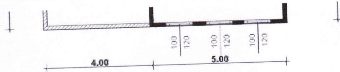
Схема второго этажа дома, размером 6,0х9,0 м + (3,0х5,0) м - каркасная веранда + (3,0х4,0) м - терраса, по наружным углам
