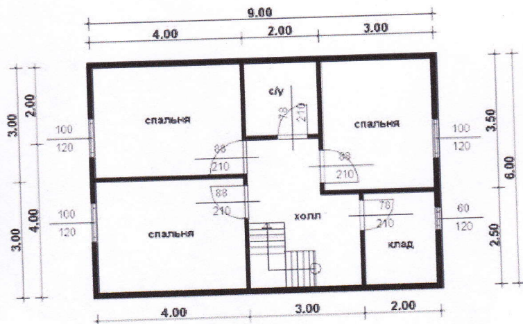
Схема второго этажа дома, размером 6,0х9,0 м + (3,0х5,0) м - каркасная веранда + (3,0х4,0) м - терраса, по наружным углам
