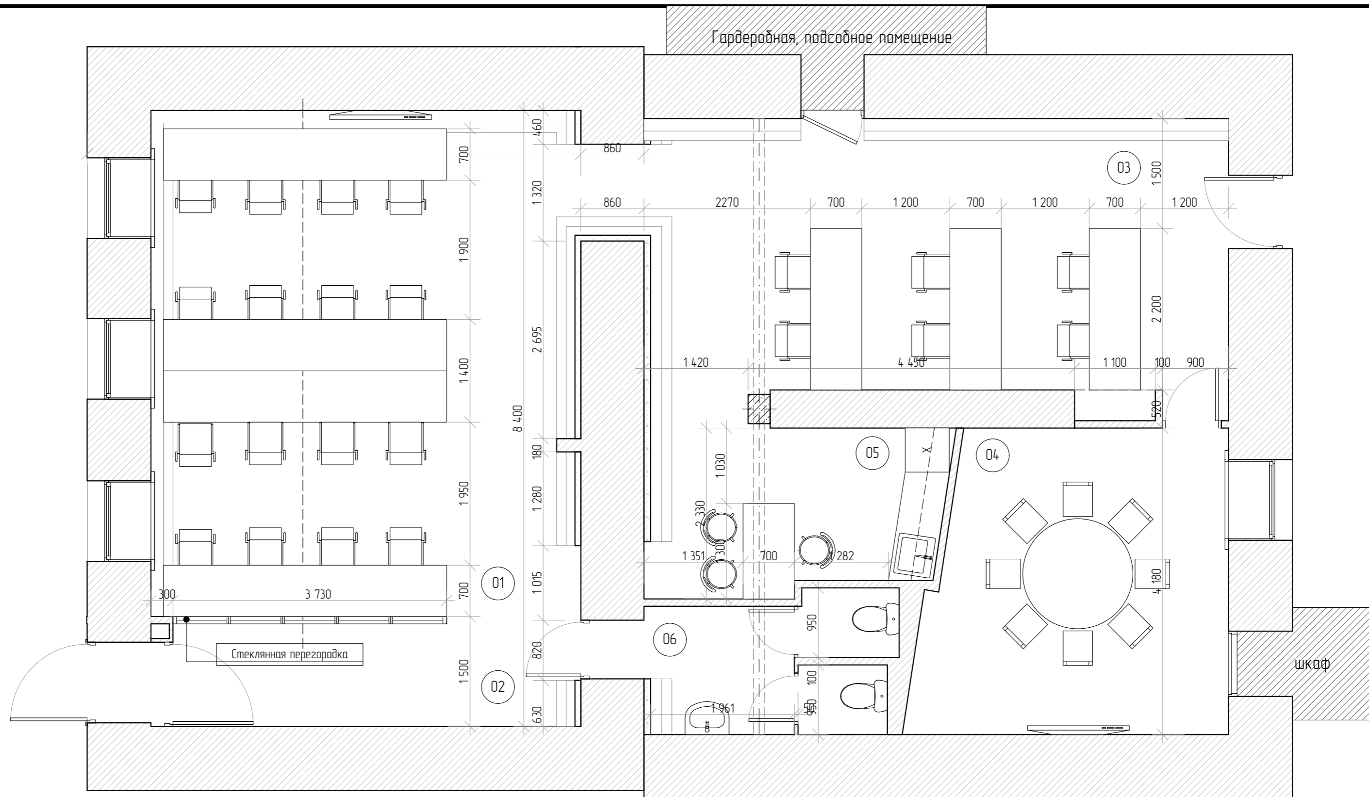
Экспликация 1-й этаж
